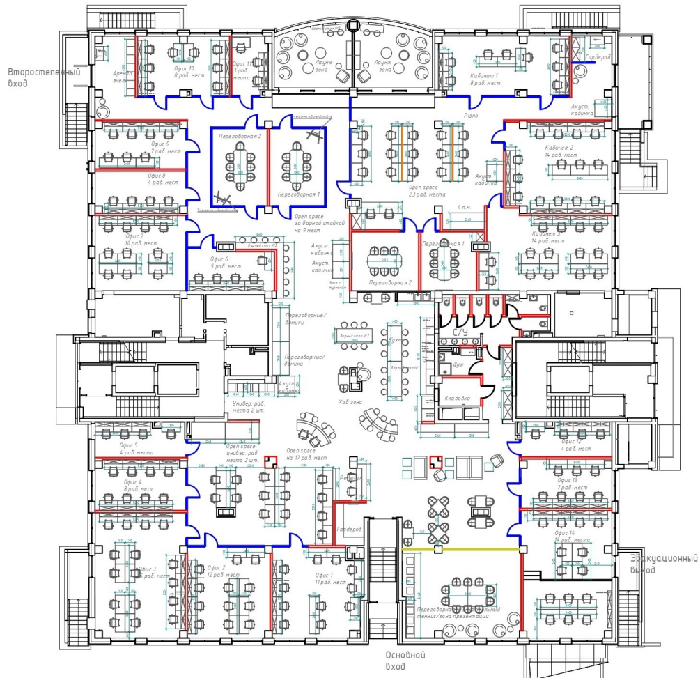
План мебели и перегородок
